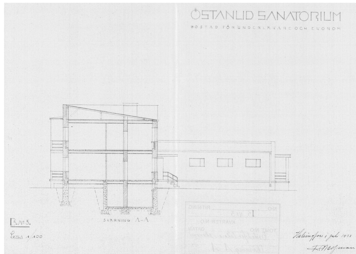
Leikkaus A-A'.
