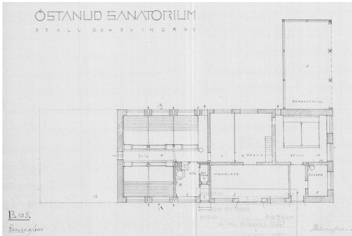
Pohjapiirros.
