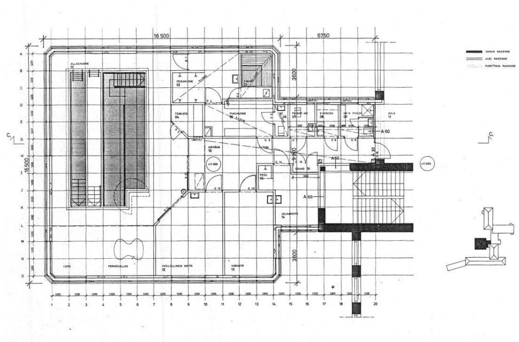
Rakennusosan D (allasosasto) pohjapiirros.
