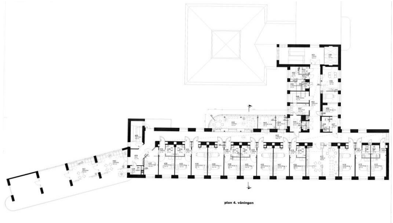
Pohjapiirros. Rakennusosan C laajennusosan muutospiirustukset.
