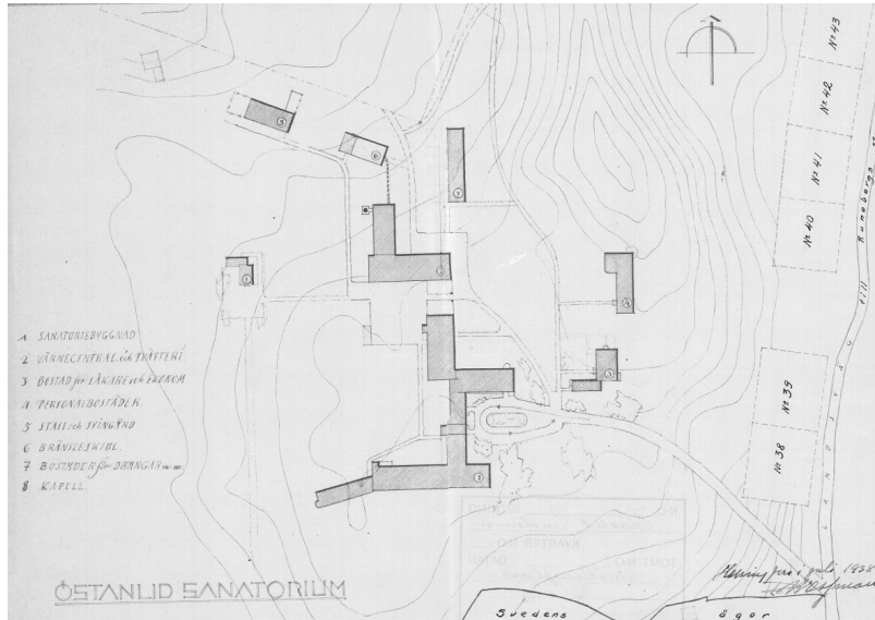
Alkuperäinen asemapiirros vuodelta 1938.
