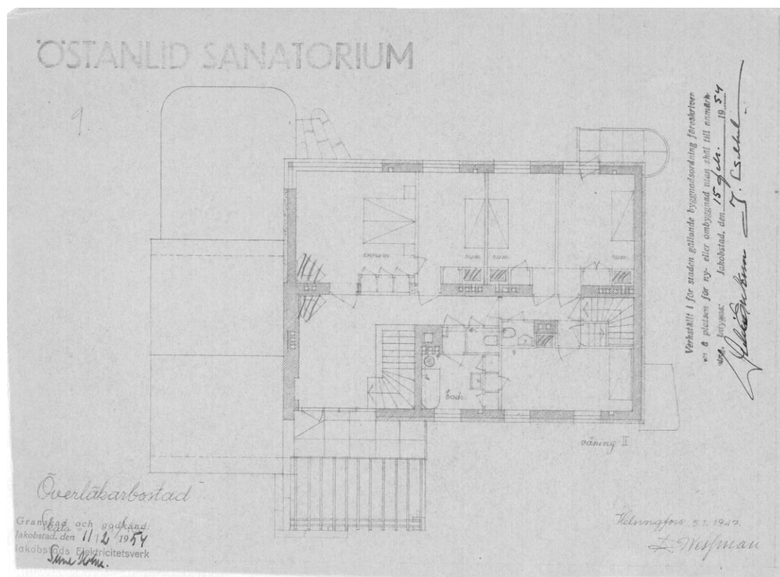
Pohjapiirros, II kerros.
