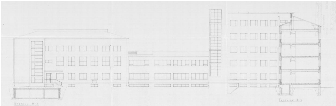
Läntinen julkisivu.
