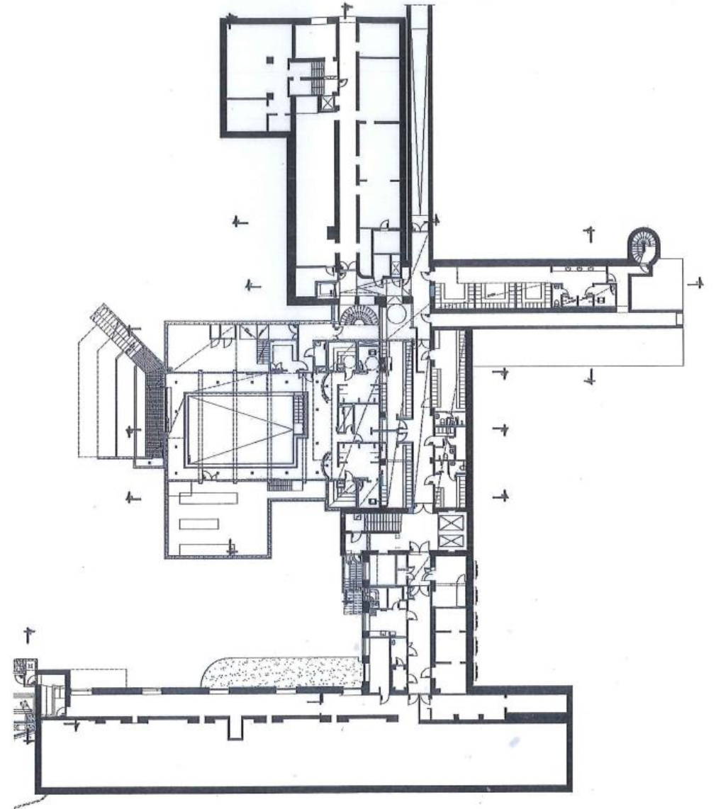
Pohjapiirros, kellarikerros
