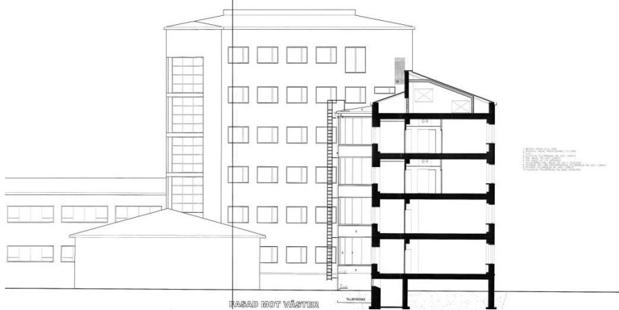
Läntinen julkisivu (leikkaus). Rakennusosan C laajennusosan muutospiirustukset.
