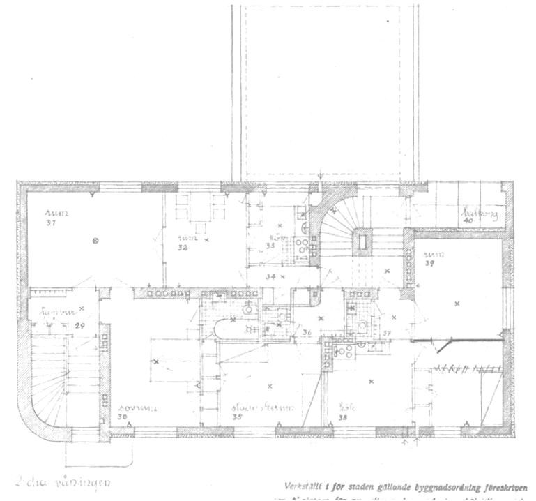
Pohjapiirros, 2 kerros.
