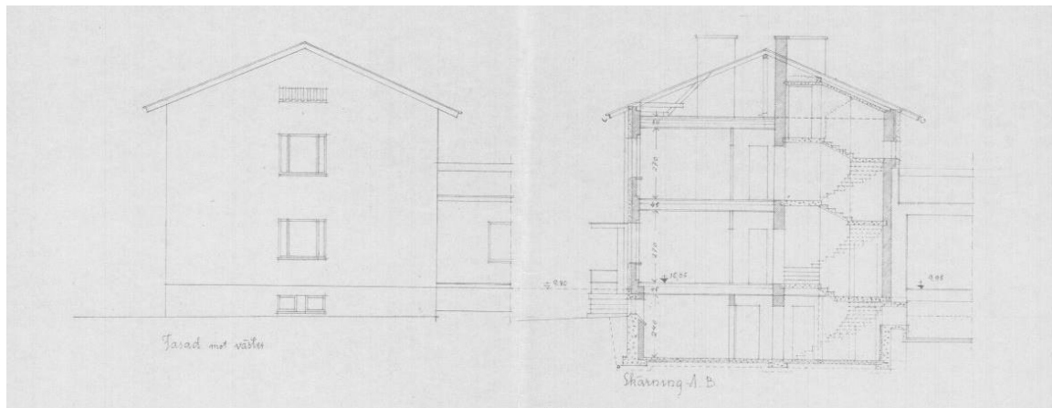
Läntinen julkisivu ja leikkaus B-B'.
