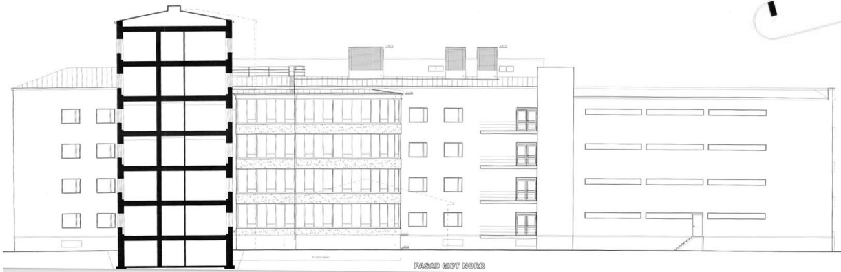
Pohjoinen julkisivu (leikkaus). Rakennusosan C laajennusosan muutospiirustukset.
