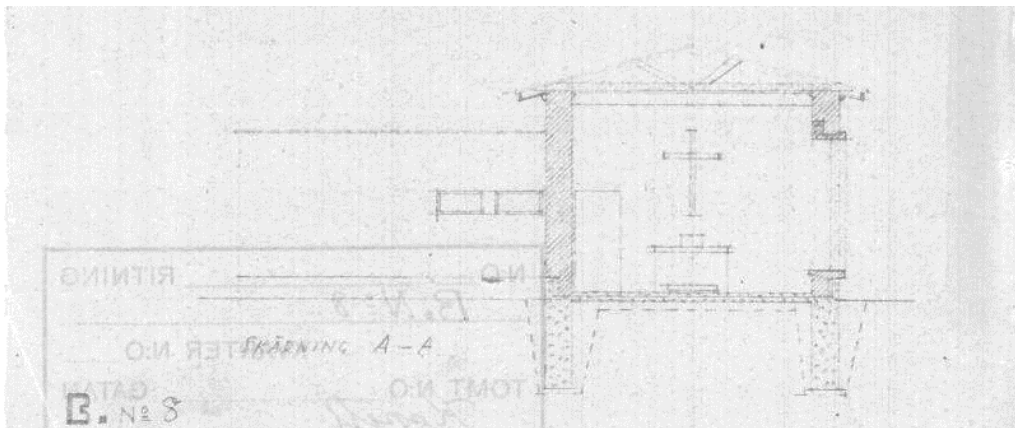
Leikkaus A-A'.
