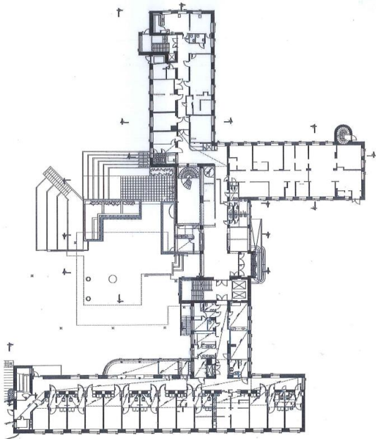
Maantasokerros.
