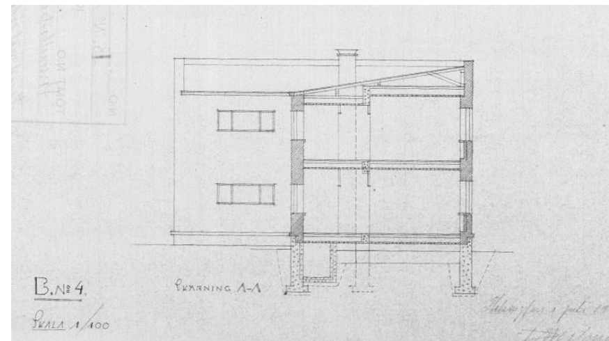
Leikkaus A-A'.
