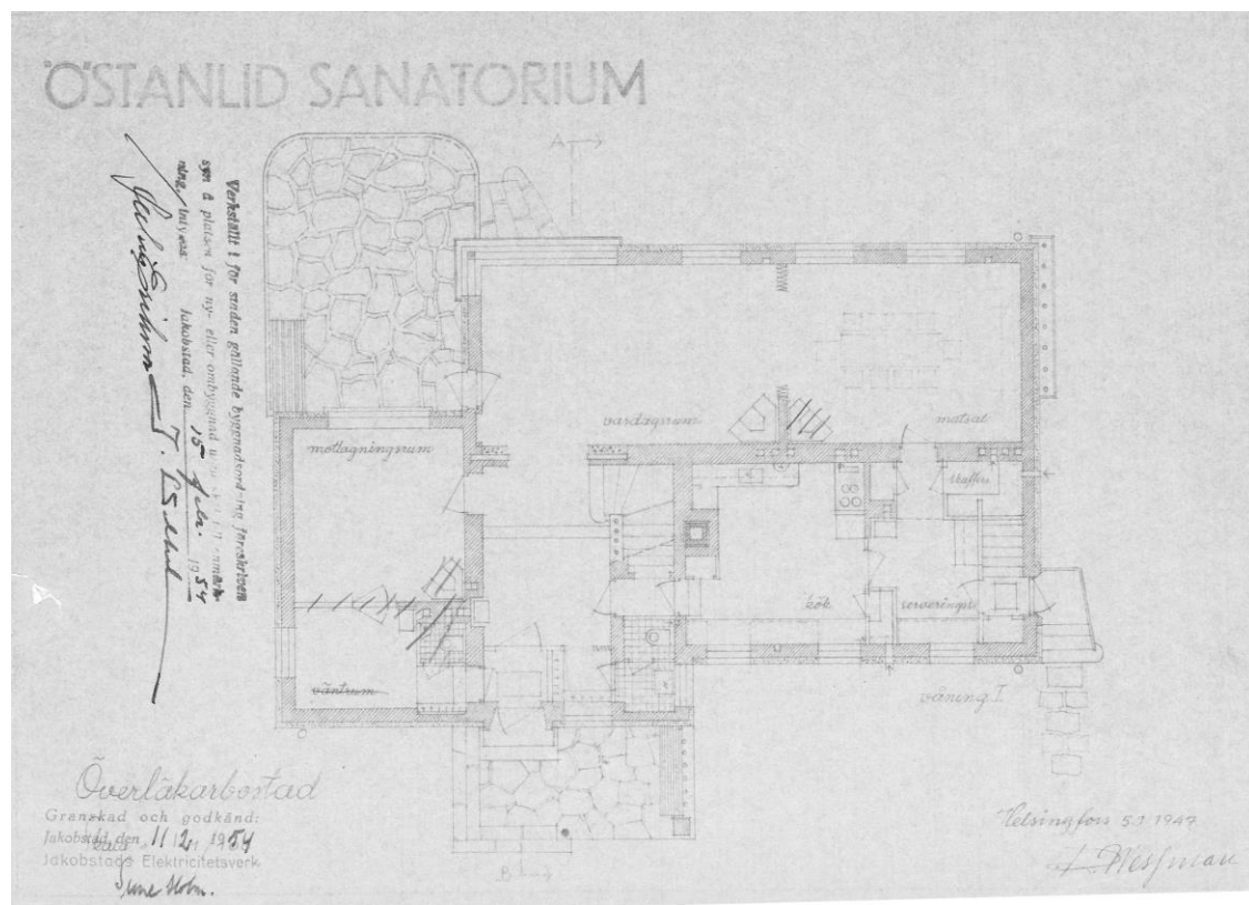
Pohjapiirros, I kerros.
