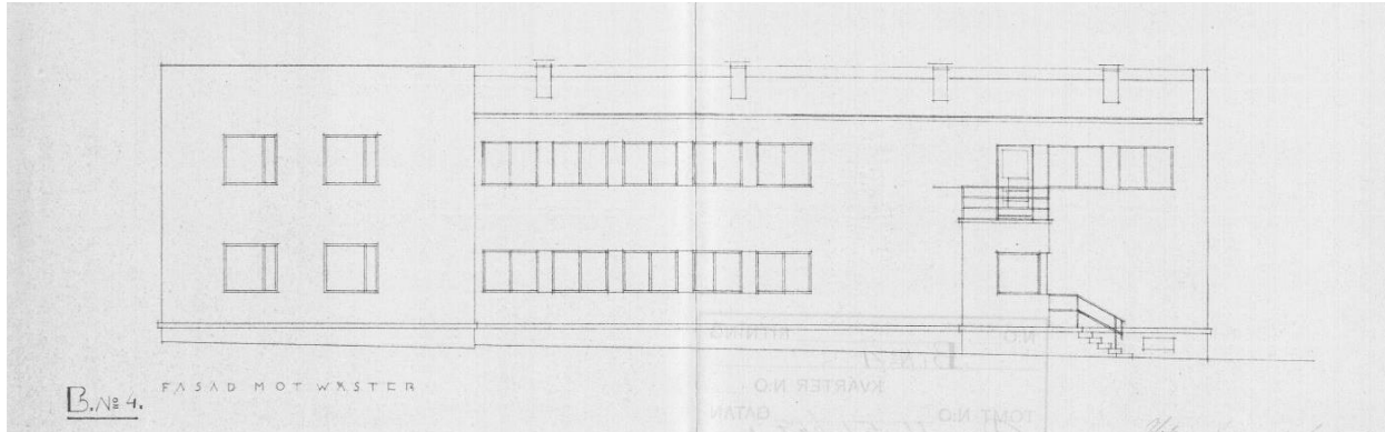
Läntinen julkisivu.
