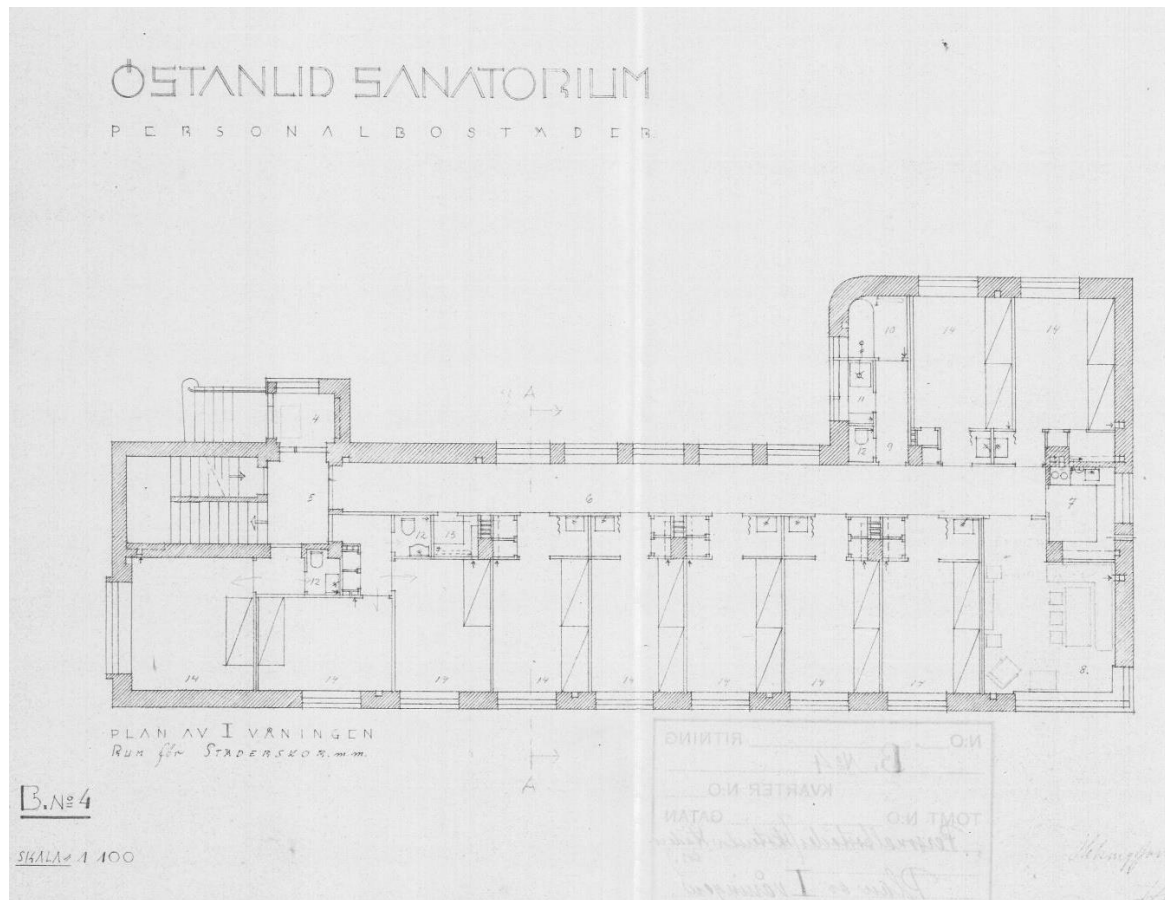
Pohjapiirros, I kerros.
